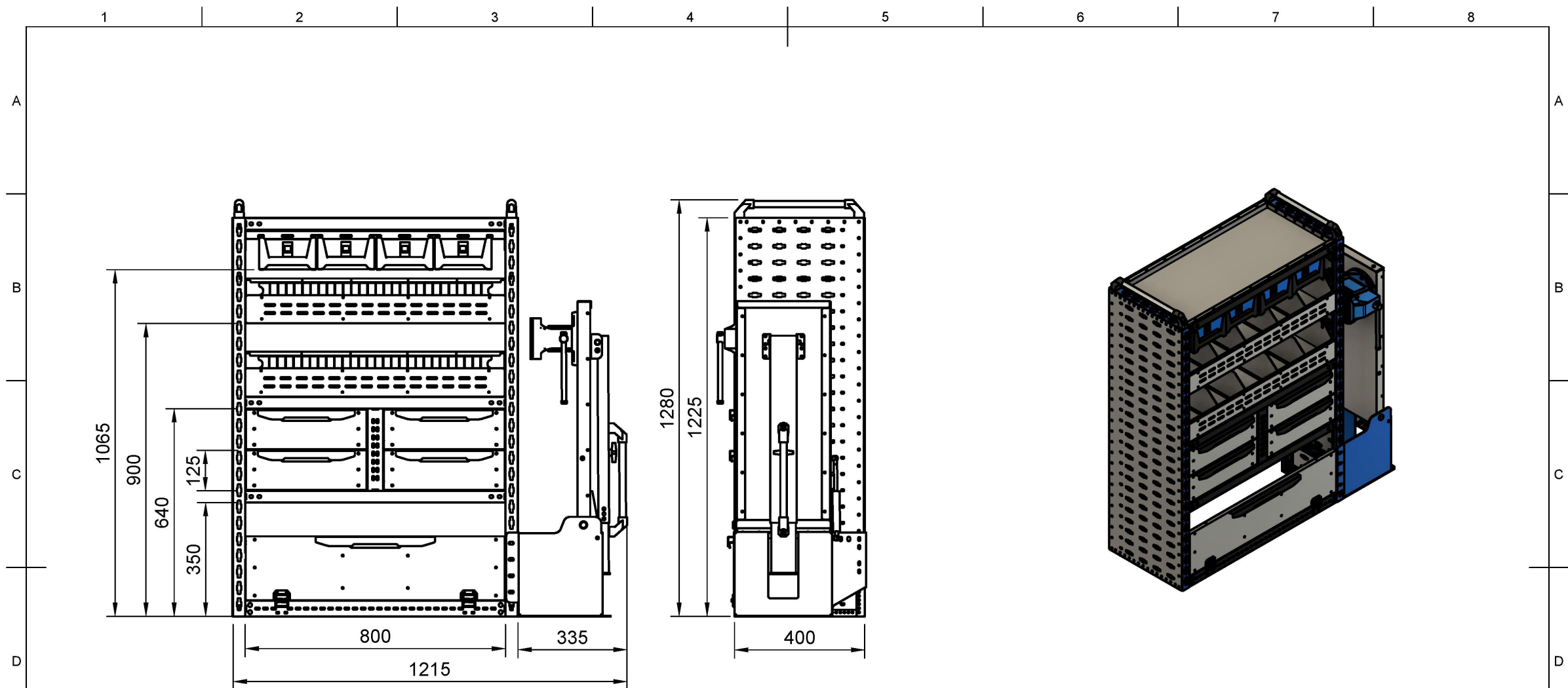
Спецификация-СВ-99.1240.12-21 Модуль 1215x400 Н1280 РЕ ПБ21
