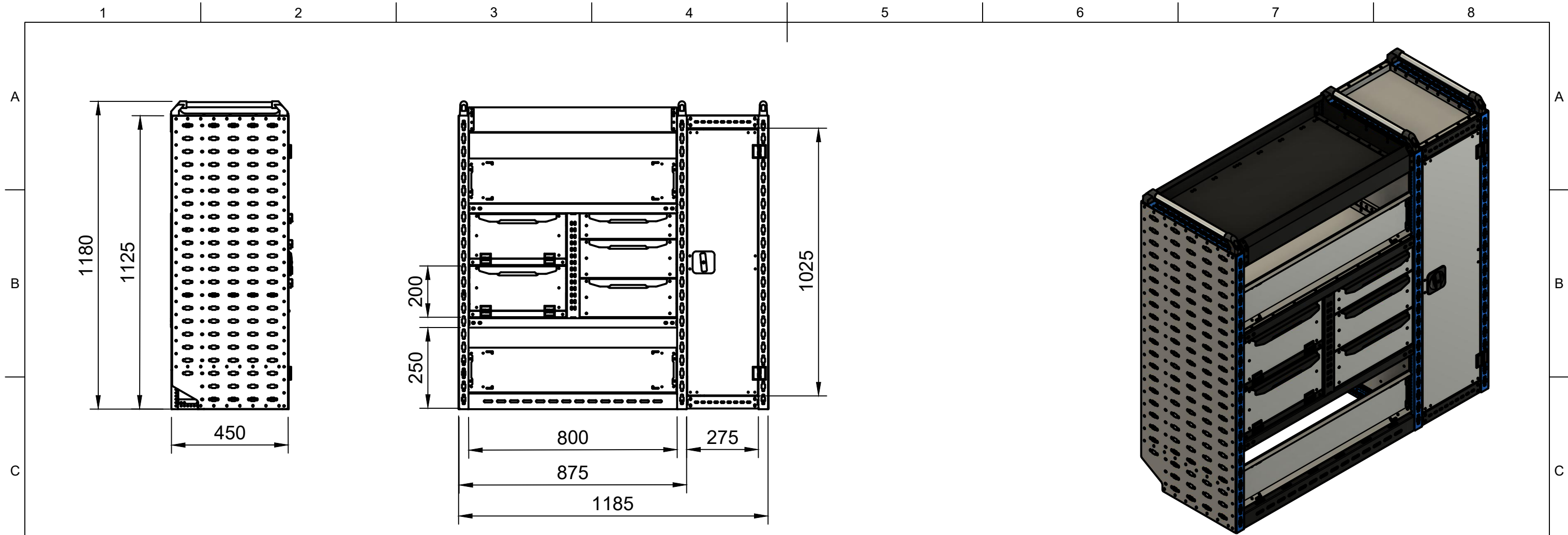
Спецификация-СВ-99.1145.11-11 Модуль 1190x450 Н1180 РЕ ЛБ11
